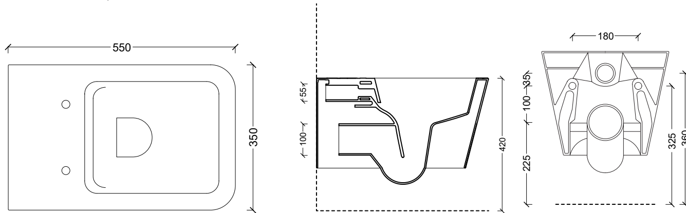
31210101 Vaso sospeso HIDE SQUARE
