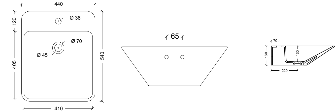
26100301 Lavabo EDGE 44X44
