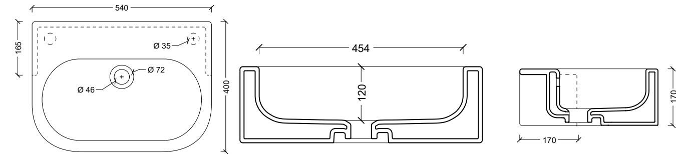
22110501 Lavabo FORM SEMINCASSO 54
