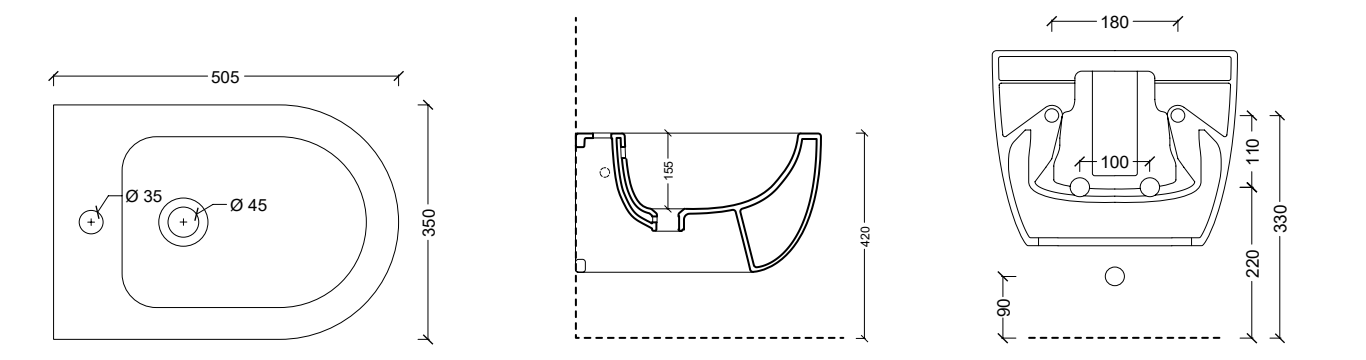
32230101 Bidet sospeso UNICA 50
