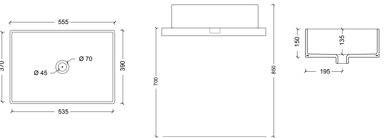
29190101 Lavabo JOKER RETTANGOLARE
