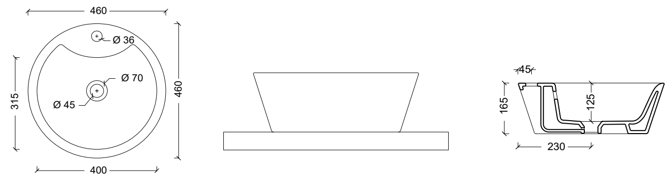
25110301 Lavabo QUADRO PLUS
