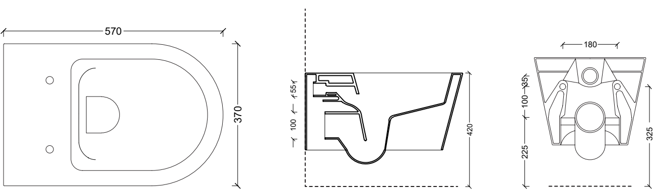
31170101 Vaso sospeso HIDE ROUND
