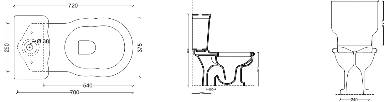
28290101 Vaso Monoblocco BOHEME scarico a parete
