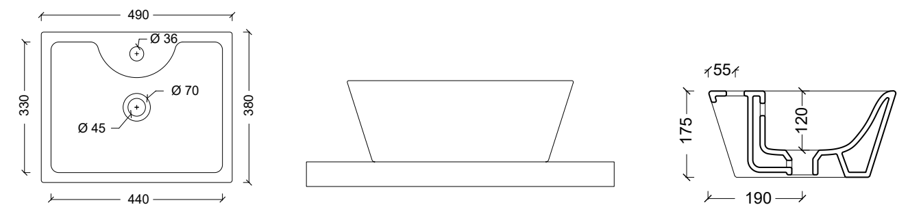
24110301 Lavabo TULIP BIG
