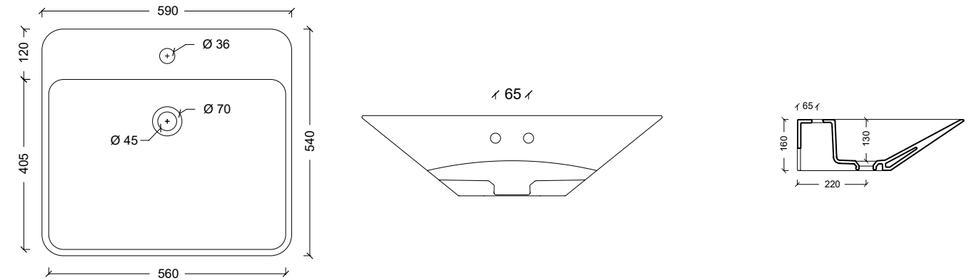
26200101 Lavabo EDGE ROUND
