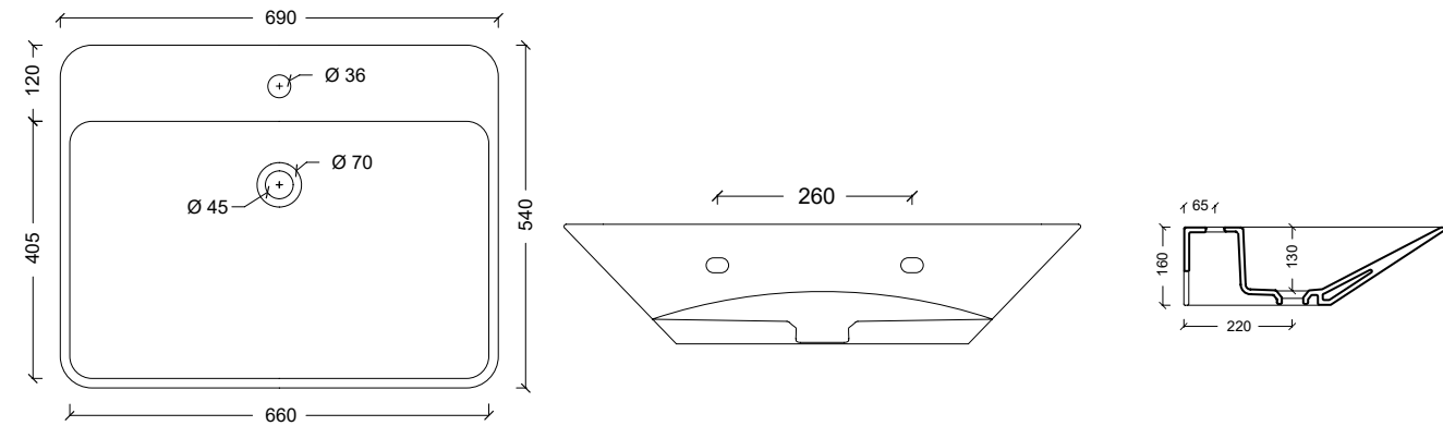
26110401 Lavabo EDGE 69X54 THIN
