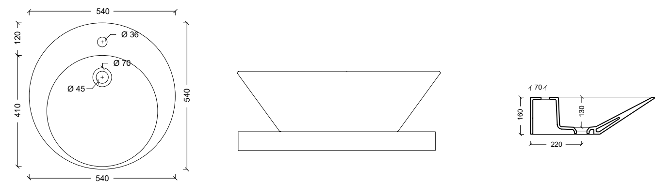
26120101 Lavabo EDGE 44X54
