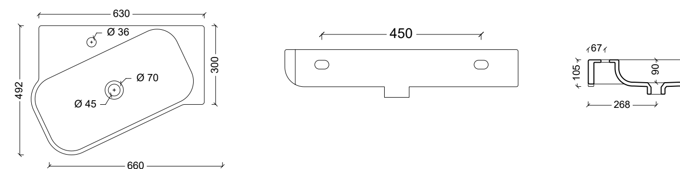
23120101 Lavabo NEAT OBLIQUO
