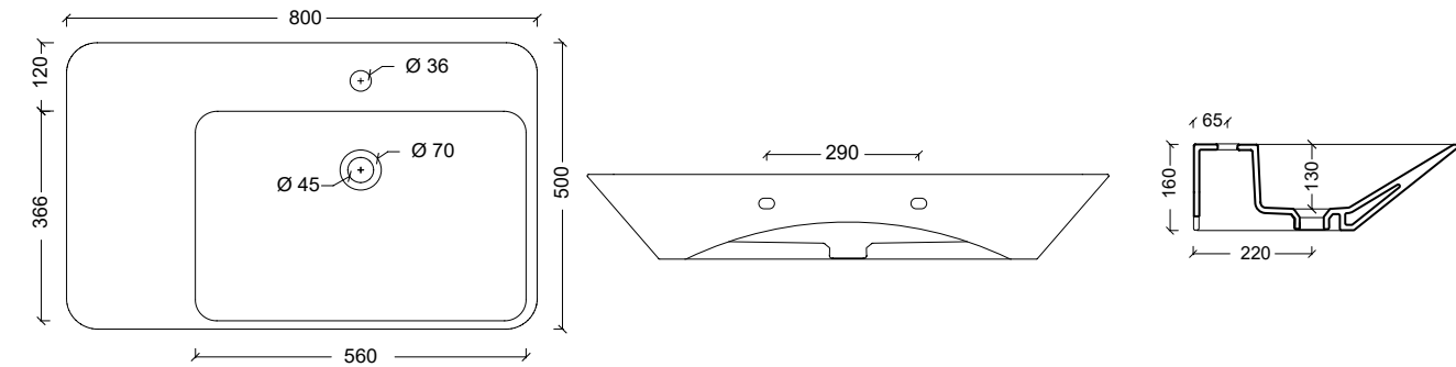
26160101 Lavabo EDGE 80X50
