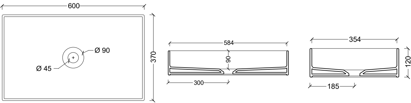
31140101 Lavabo HIDE CIRCLE
