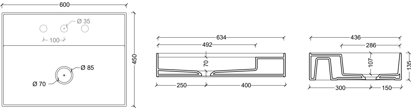
31230101 Lavabo sospeso e appoggio 60 x 45
