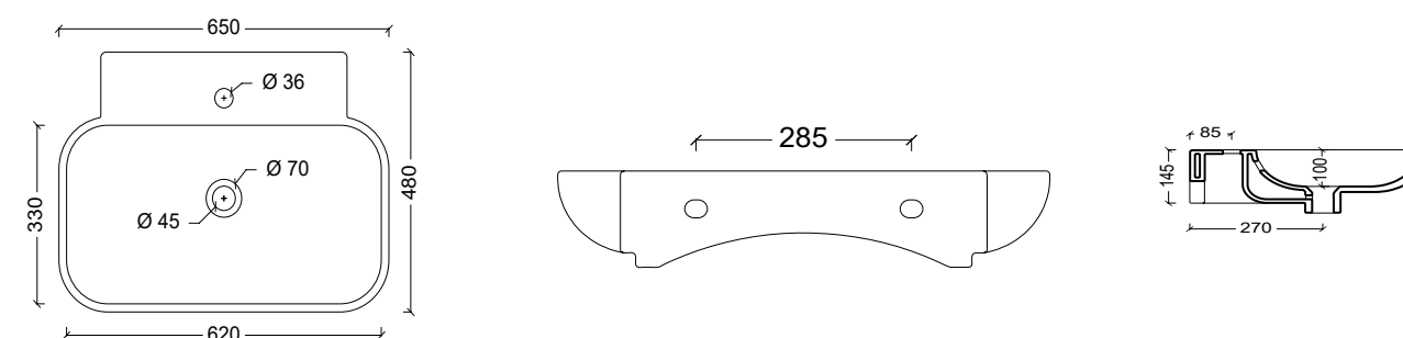
23120101 Lavabo NEAT OBLIQUO
