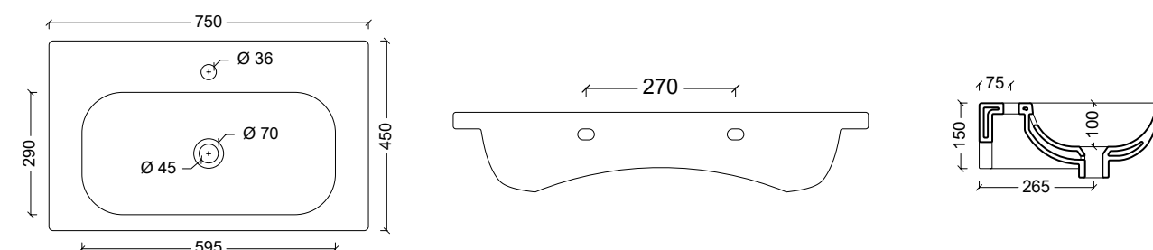
23110101 Lavabo NEAT EASY
