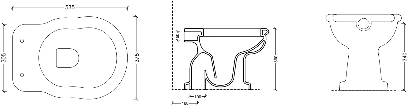
28210101 Vaso a terra BOHEME scarico a parete
