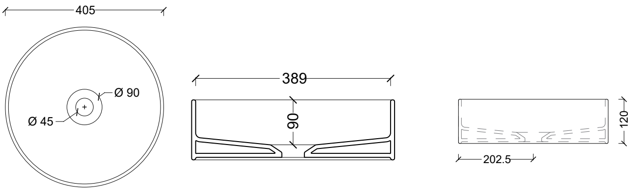
31140101 Lavabo HIDE CIRCLE
